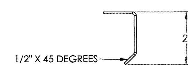
45/90 EDGE DETAIL
